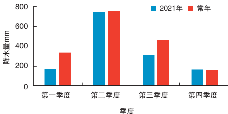
2021年韶关市各季度降水量
