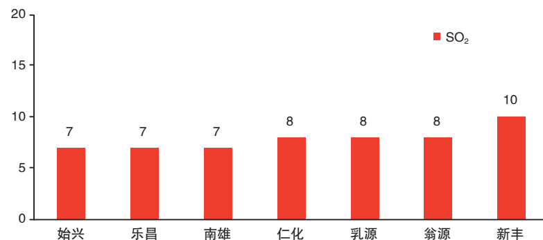
各县(市)城区 SO 2 年均值比对(单位:微克/立方米)
