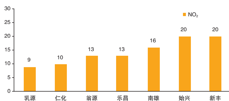
各县(市)城区 NO 2 年均值比对(单位:微克/立方米)
