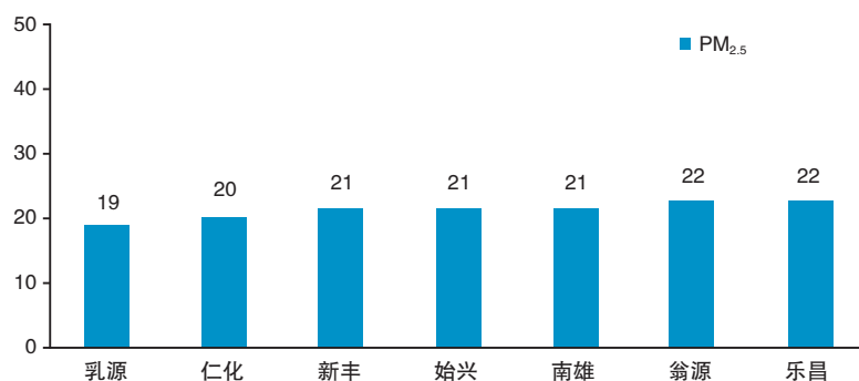
浓度 (微克/立方米)
