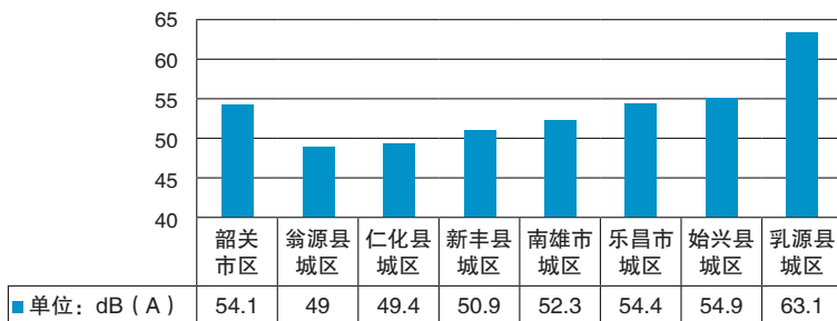
全市昼间区域声环境质量
