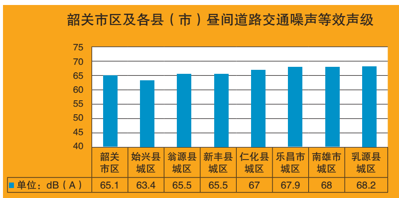
全市昼间道路交通噪声
