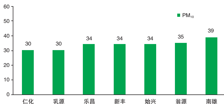
各县(市)城区 PM 10 年均值比对(单位:微克 / 立方米)
