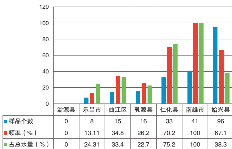
各县(市、区)酸雨统计
