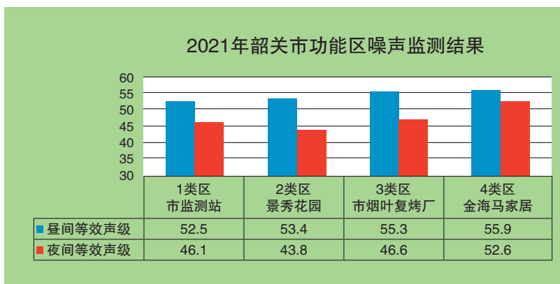
韶关市功能区噪声监测结果
