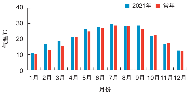
2021年韶关市各月平均气温
