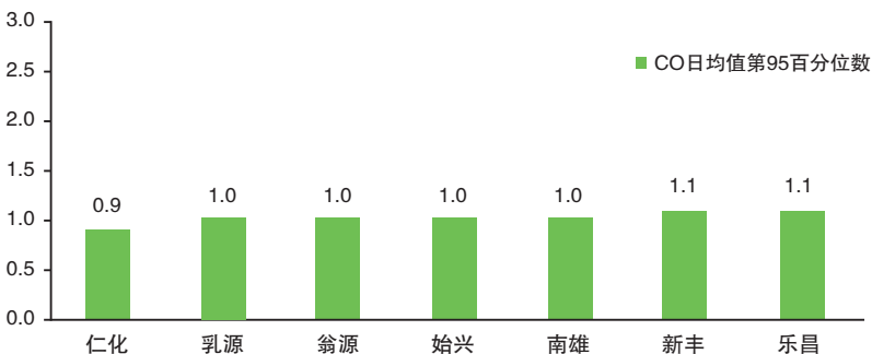
各县(市)城区 CO 日均值第 95 百分位数比对(单位:毫克 / 立方米)
