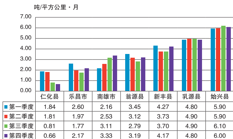
各县(市)降尘季均值
