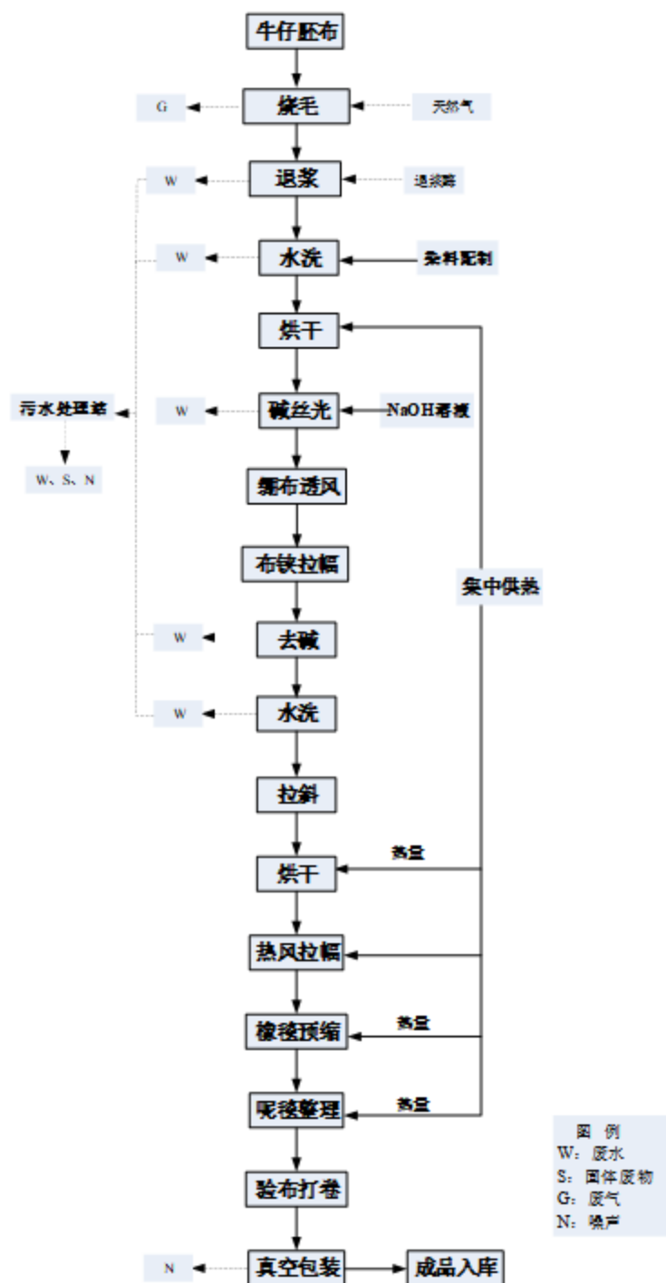
图 2-6 丝光后整理工艺流程与产污节点图
