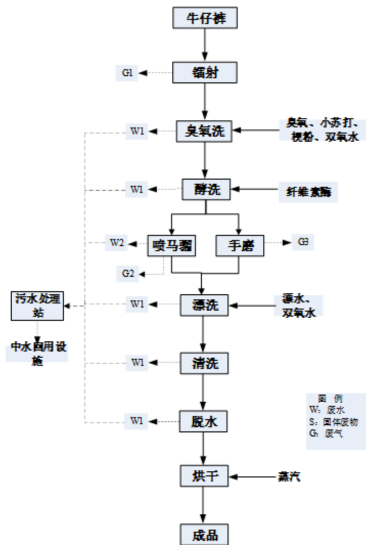
圖 2-7 牛仔褲水洗生產線工藝流程與產污節點圖
