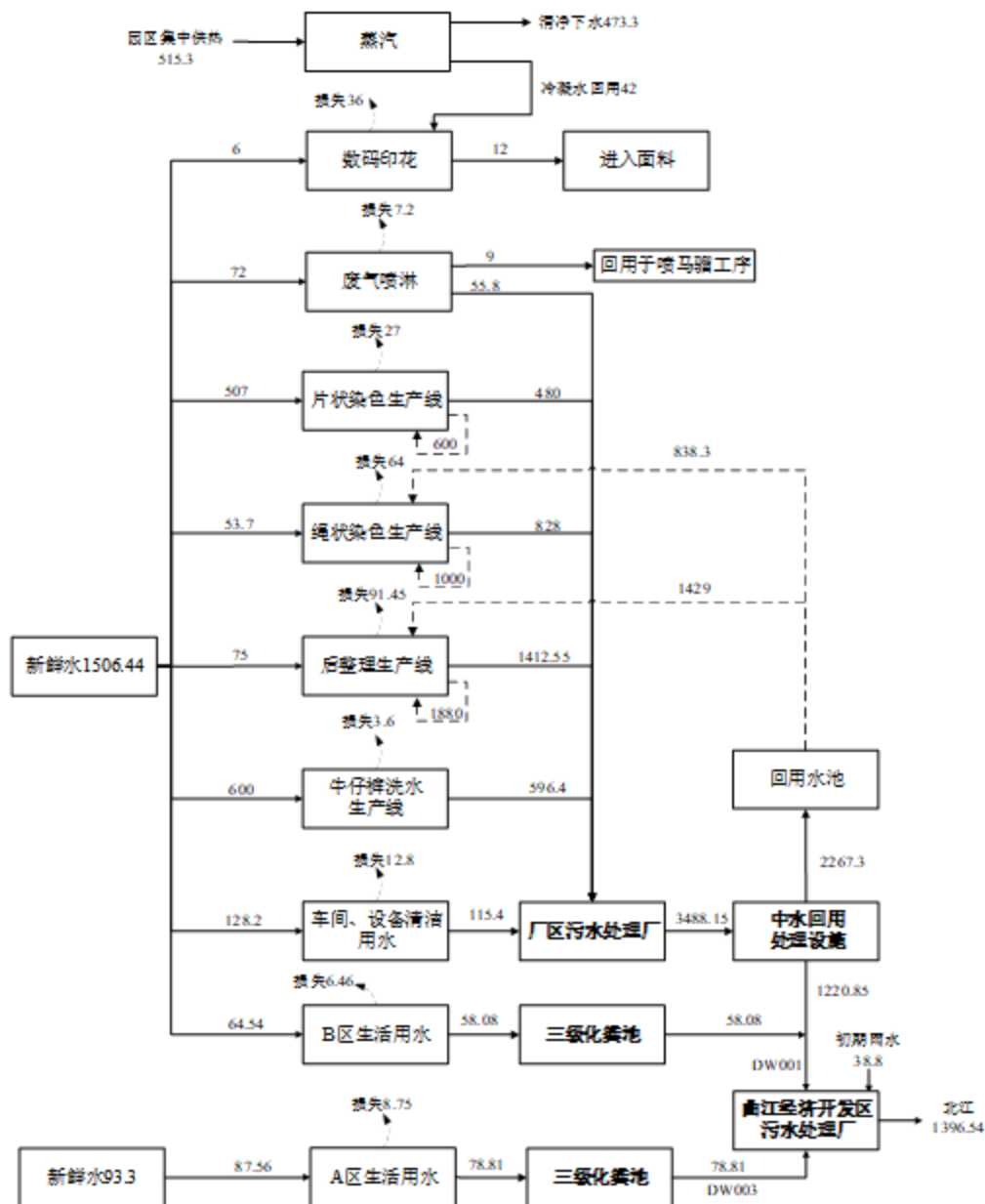
图2-2 全厂水平衡图 (m 3 /d)
