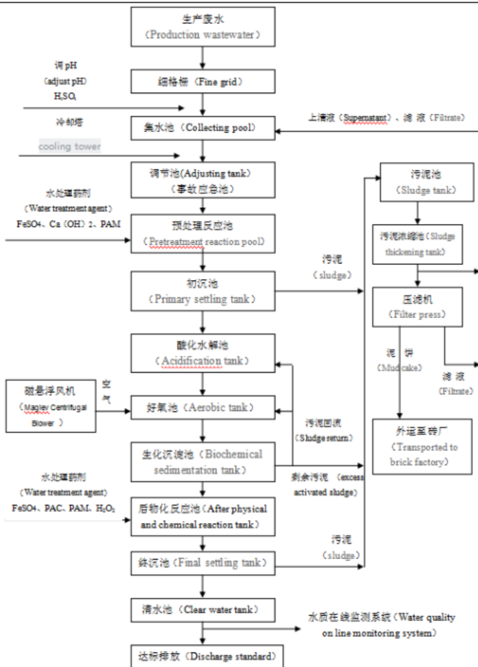
图 2-9 厂区污水处理站工艺流程图
