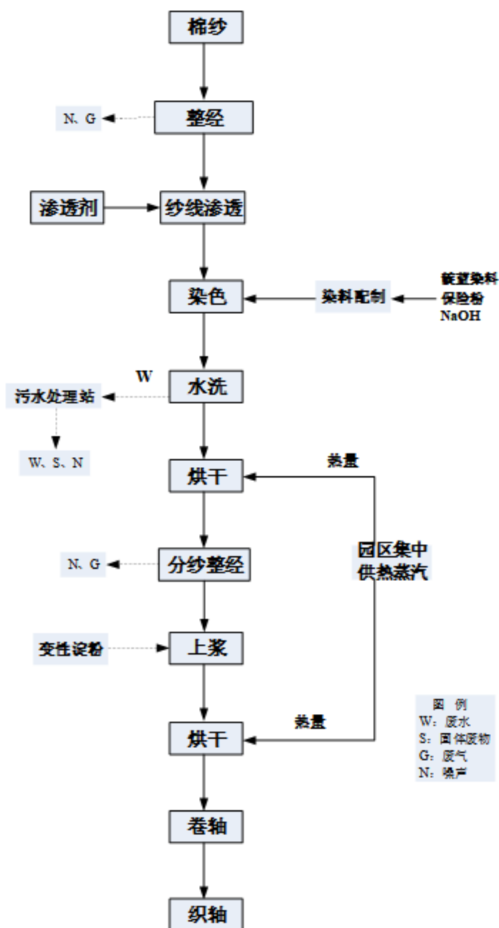
图 2-4 片状浆染生产线工艺流程与产污节点图
