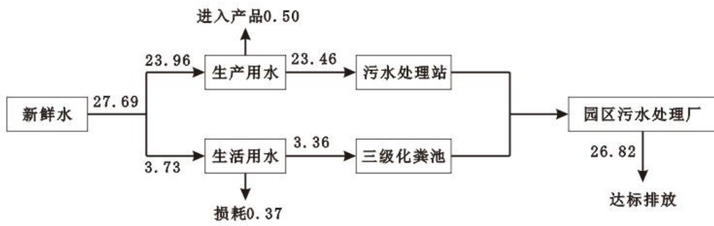
图 2-1 项目用水平衡图 (单位: \text{m}^3/\text{d} )
