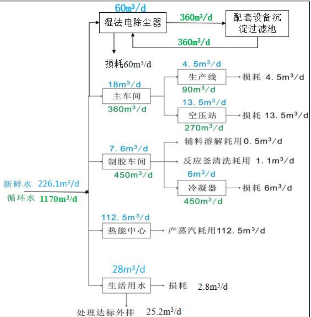
图 1 现有工程水平衡图（单位 \text{m}^3/\text{d} ）
