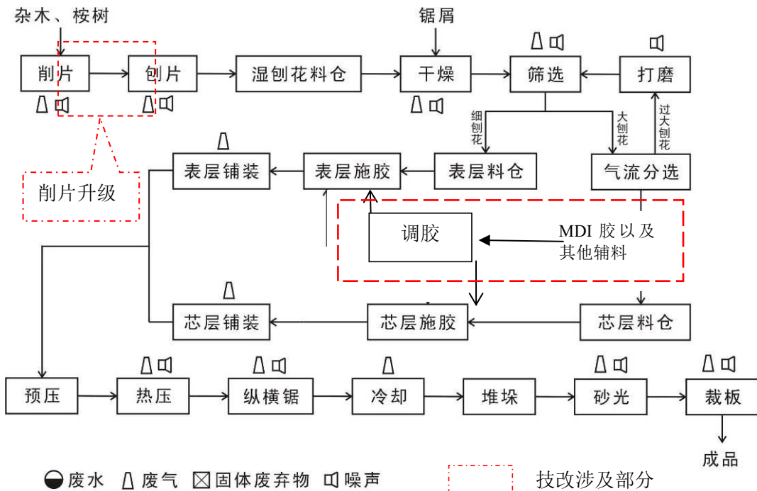
图 4 刨花板生产工艺流程及产污环节图
