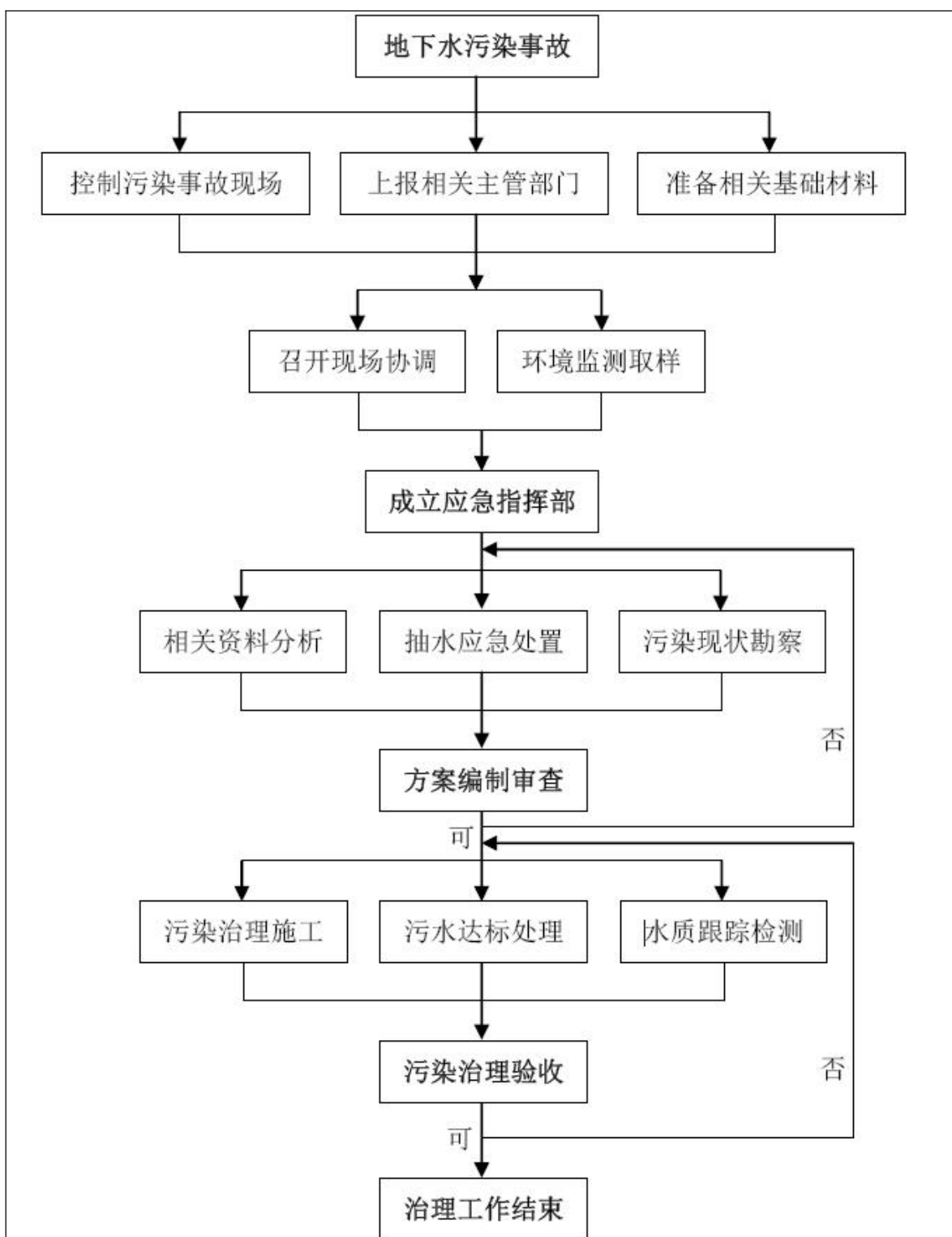
图 20 地下水污染应急治理程序图
