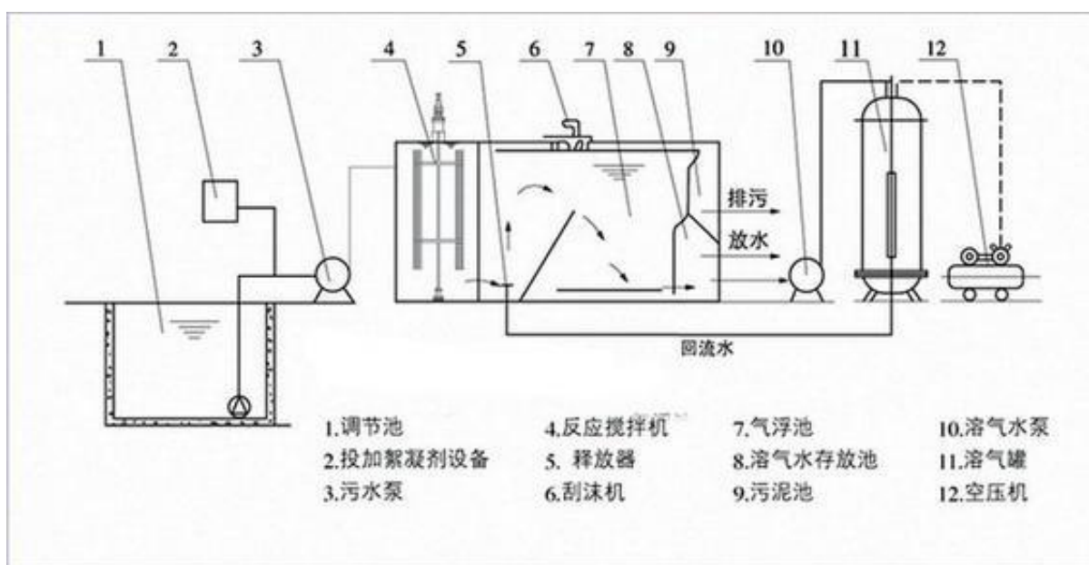
图 17 本项目生产废水处理工艺流程图
