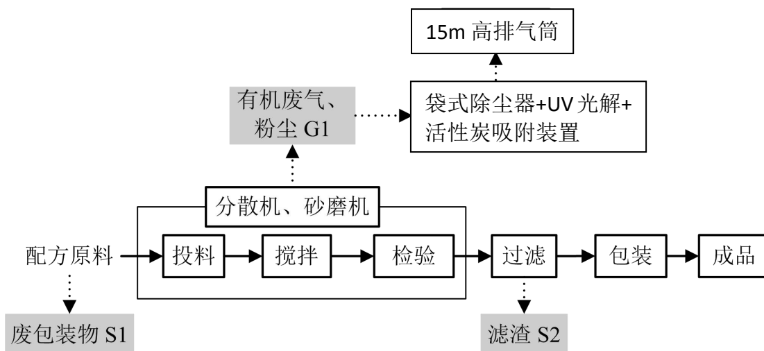
图 12 印刷油墨生产工艺流程及产污环节图
