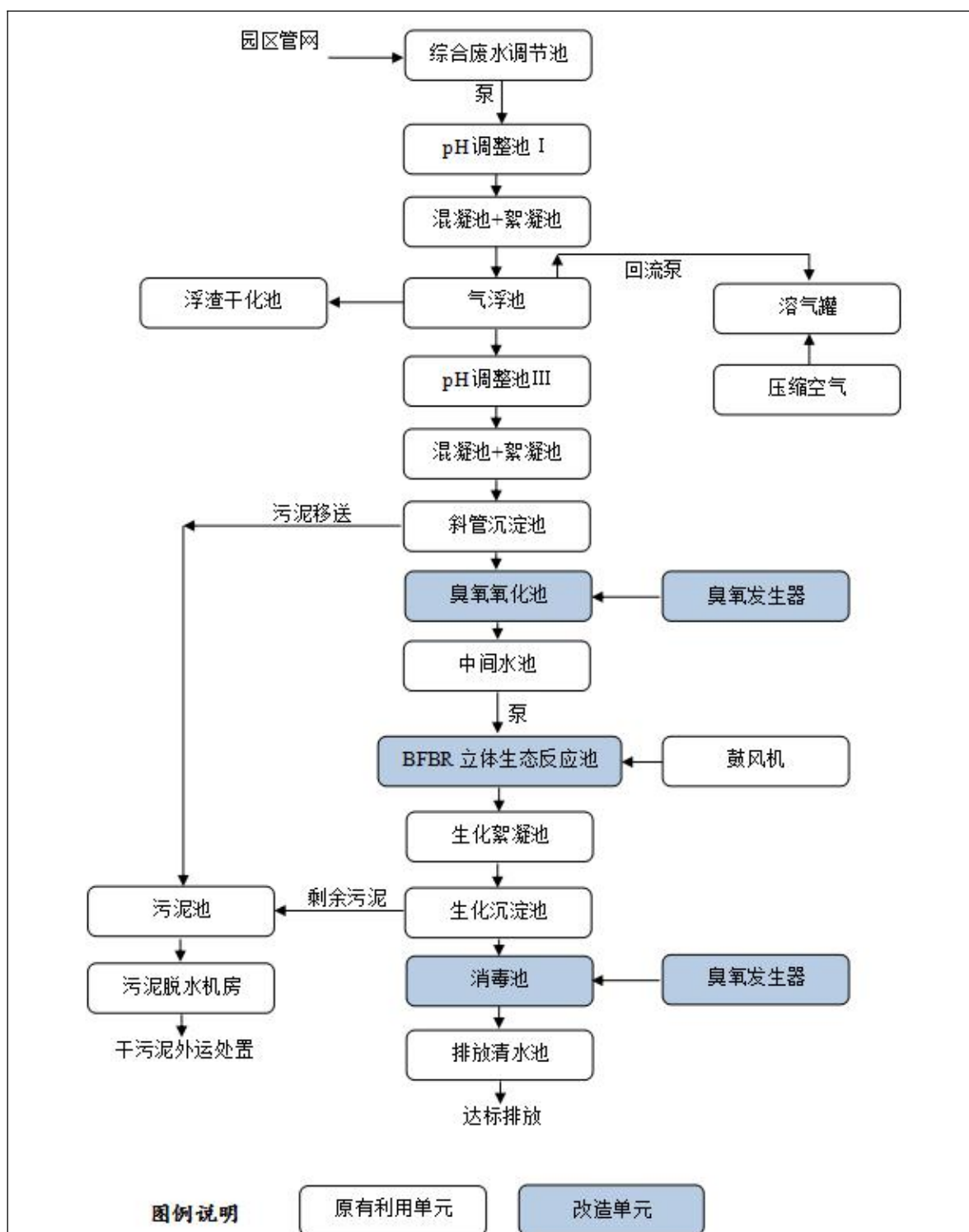
图 18 南雄市精细化工基地污水处理厂处理工艺流程图
