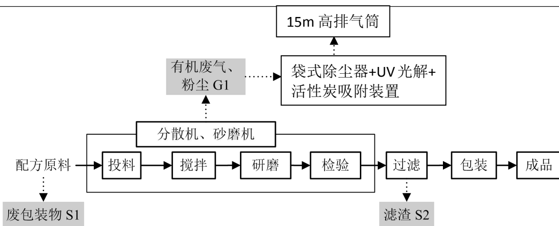
图 15 丙烯酸清烘漆生产工艺流程及产污环节图
