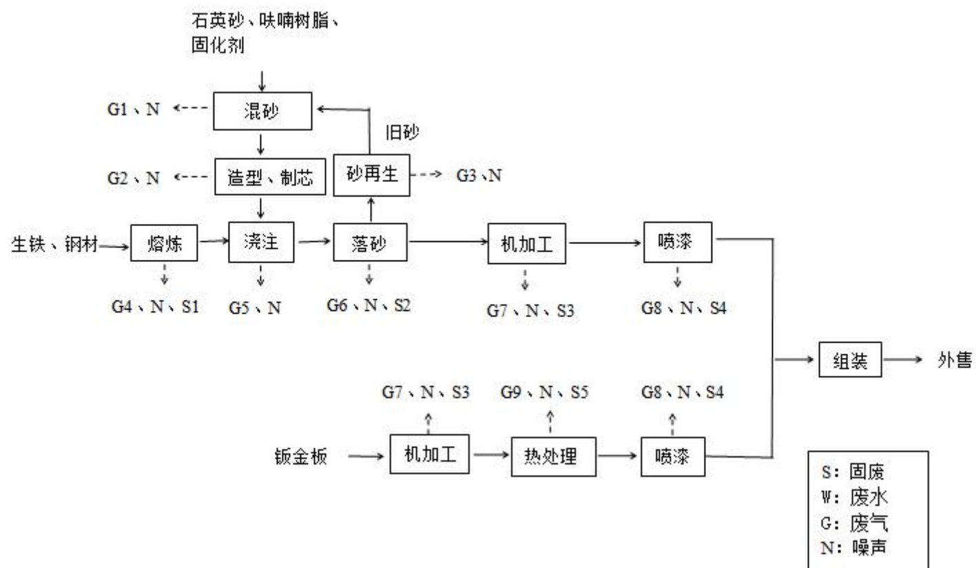
图 2-2 项目生处理产工艺流程及产污节点图
