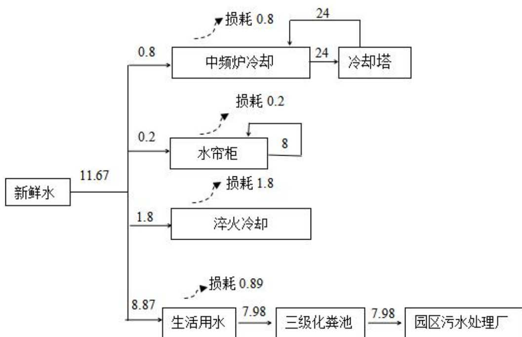
图 2-1 项目水平衡图 \text{m}^3/\text{d}
