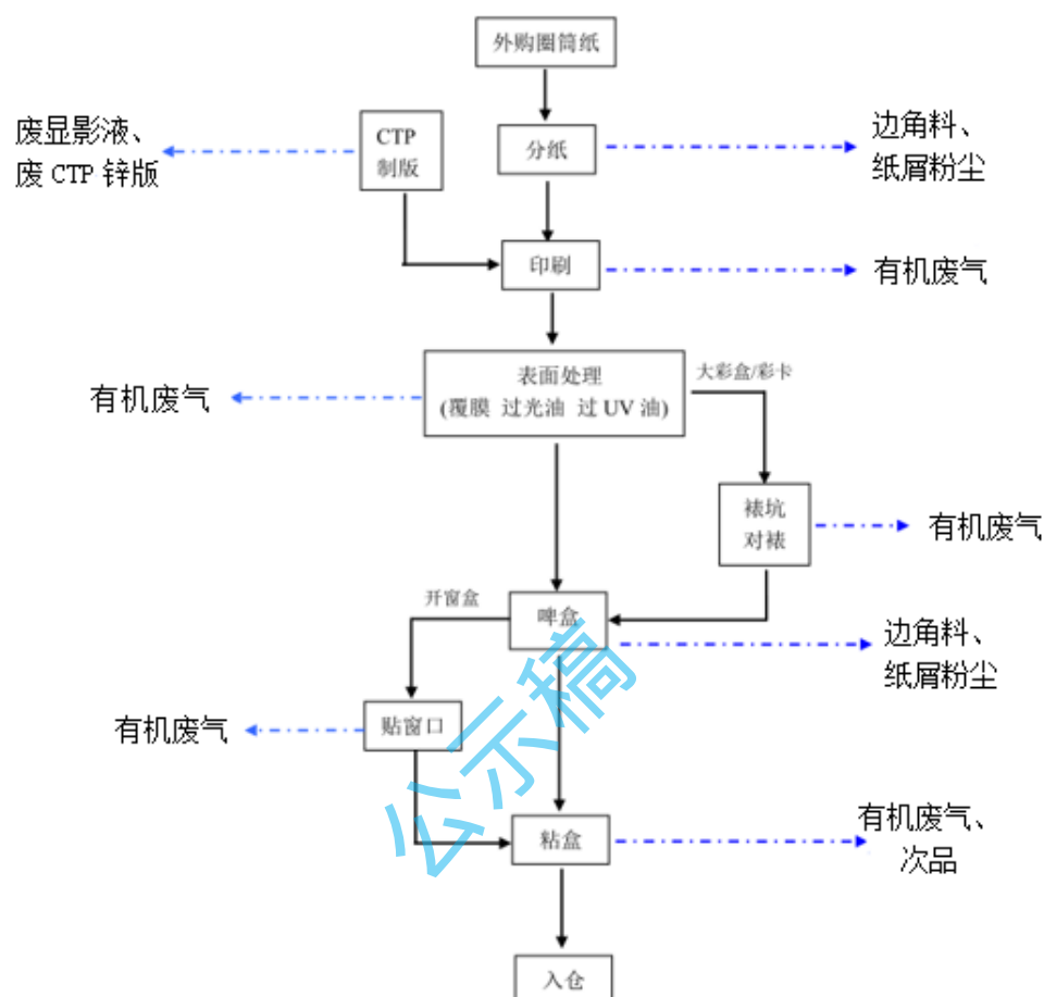
图 2-7 彩盒生产工艺流程及产污节点图
