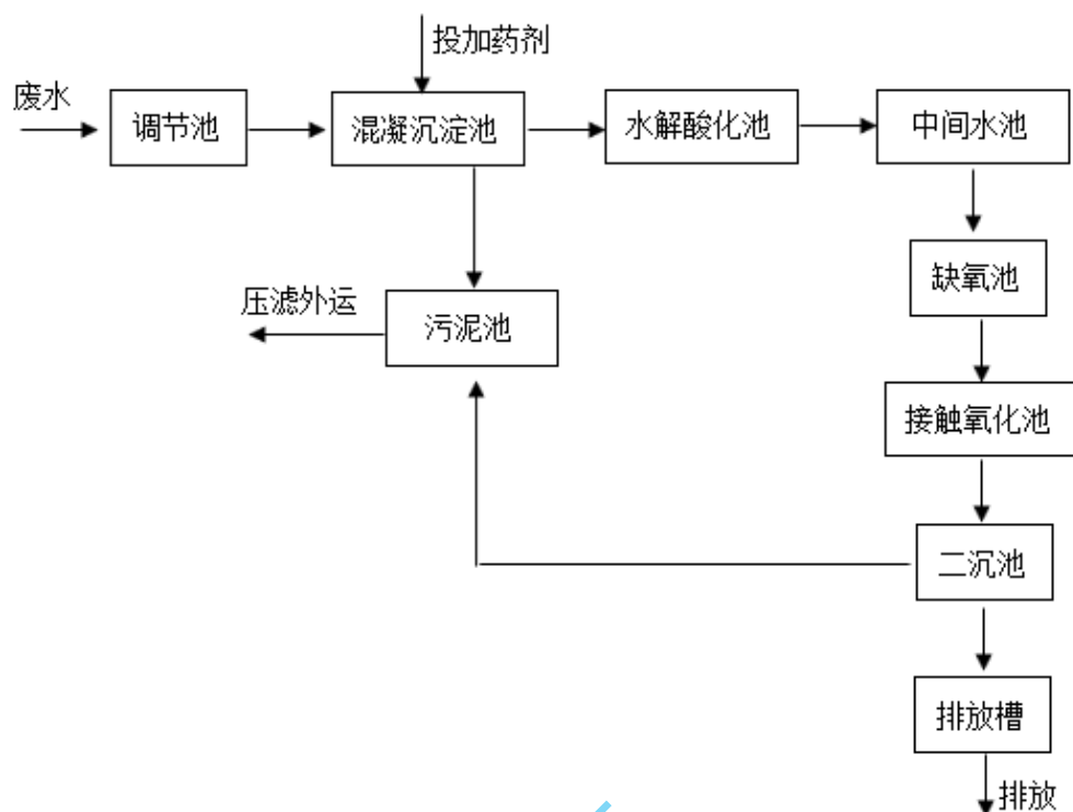
图 4-1 污水处理站污水处理工艺流程图
