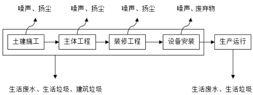
图 2-6 施工期工艺流程及产污节点图
