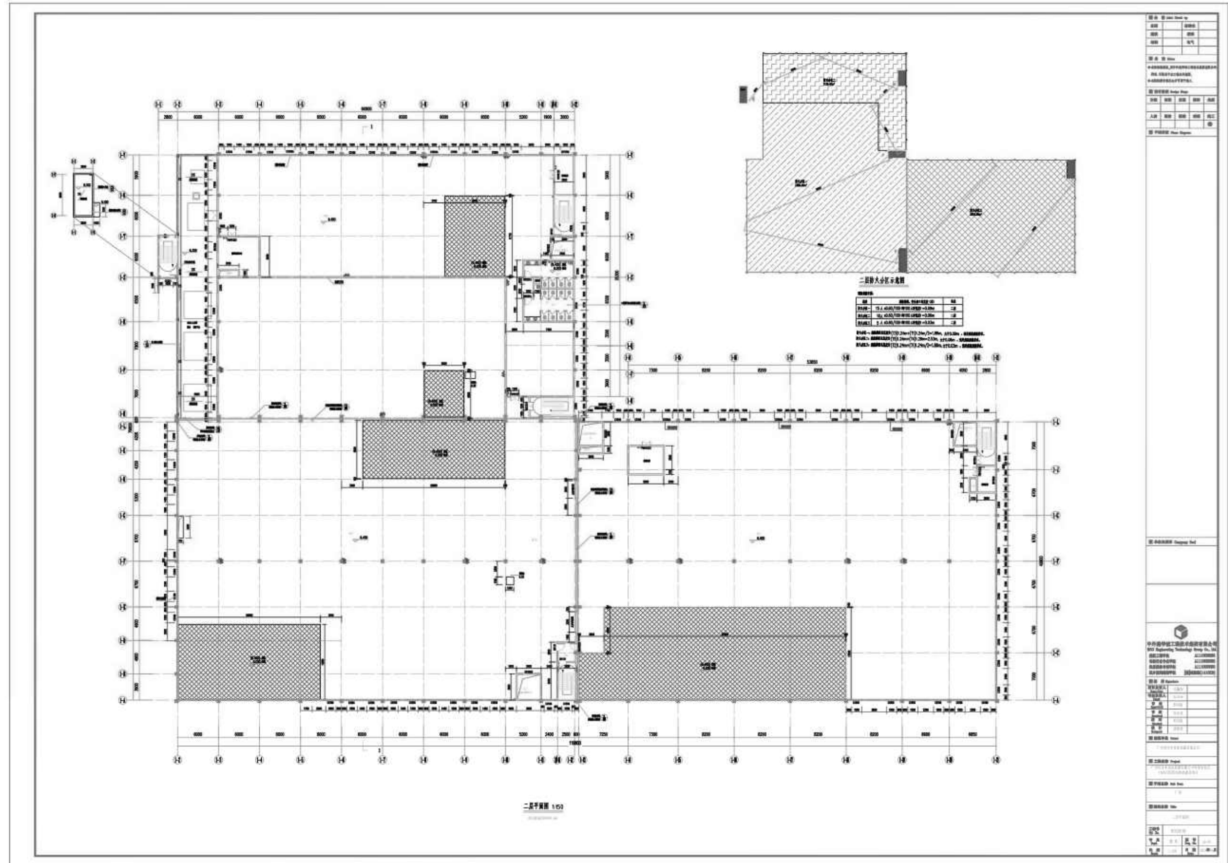
图 3-7 加工车间二层平面布置图
