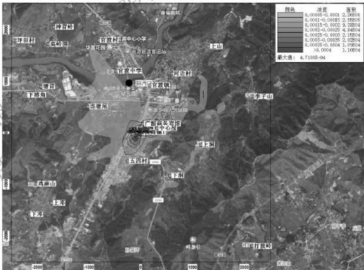
图 5-8 正常排放情况下 PM 10 日平均浓度最大值分布图
