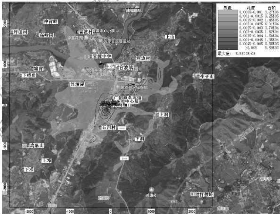
图 5-6 正常排放情况下 NO 2 日平均浓度最大值分布图
