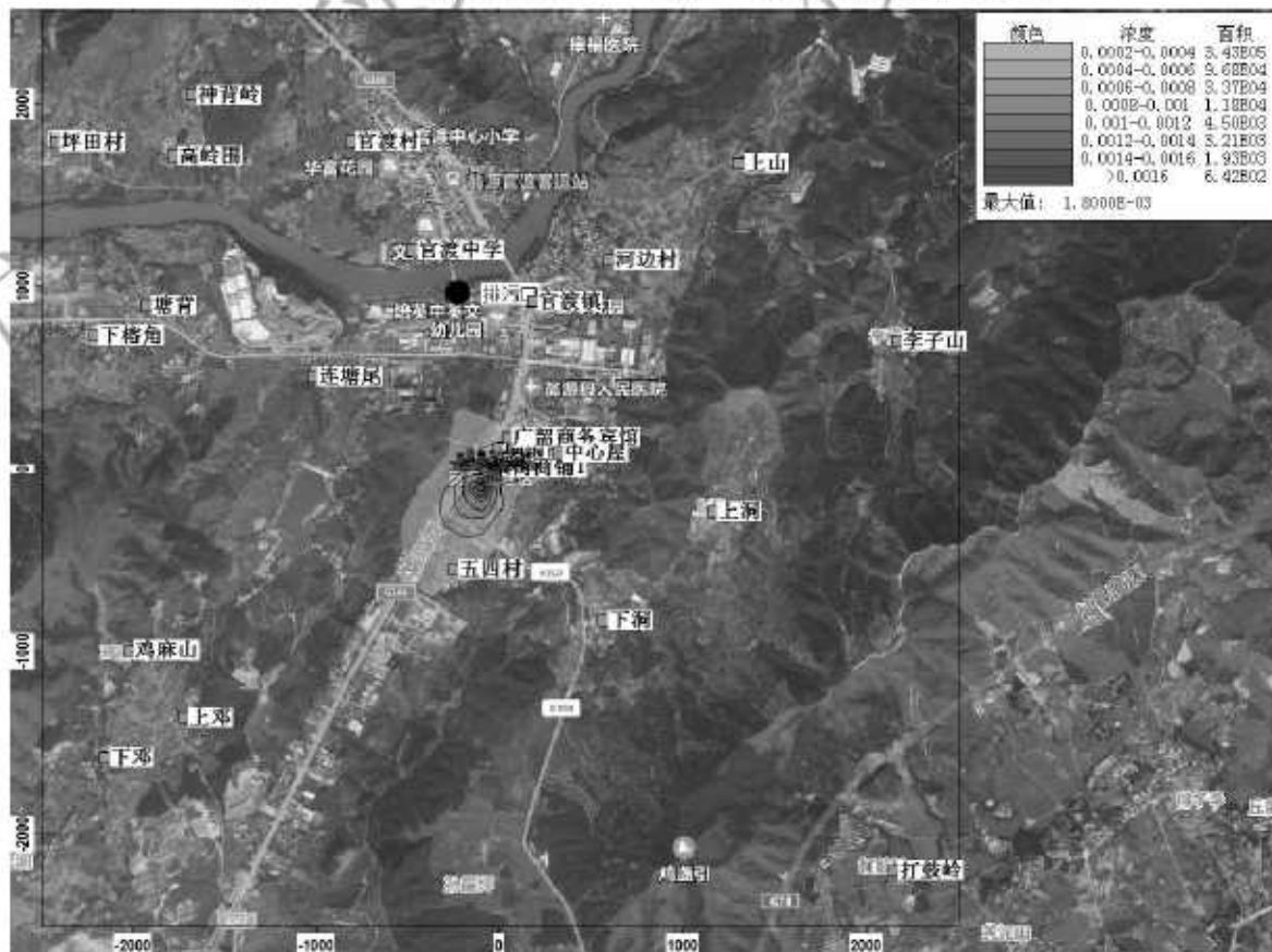
图 5-7 正常排放情况下 NO 2 年平均浓度最大值分布图
