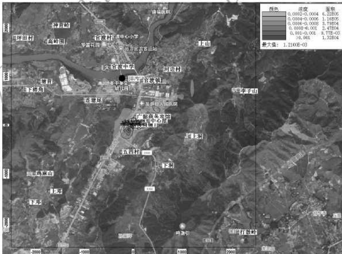
图 5-3 正常排放情况下 SO 2 日平均浓度最大值分布图
