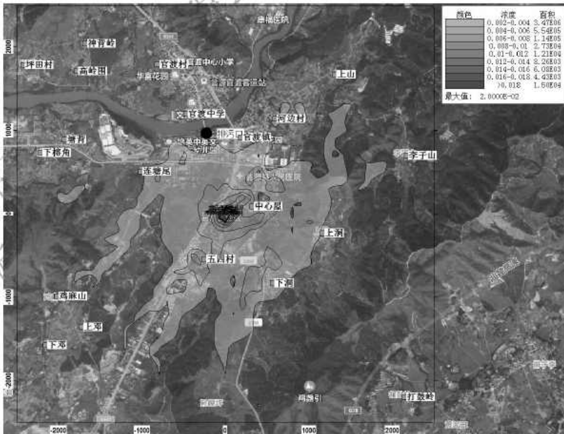
图 5-14 非正常排放情况下 NH 3 小时平均浓度最大值分布图
