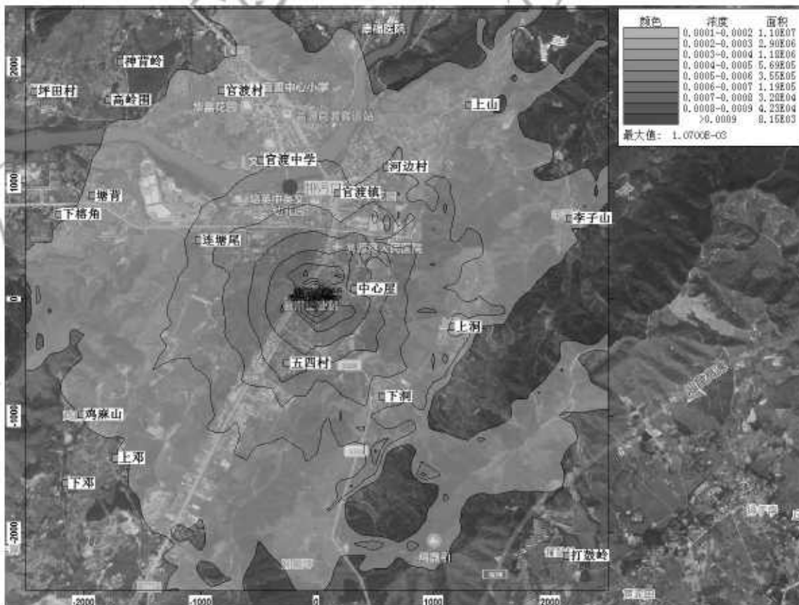
图 5-15 非正常排放情况下 H 2 S 小时平均浓度最大值分布图
