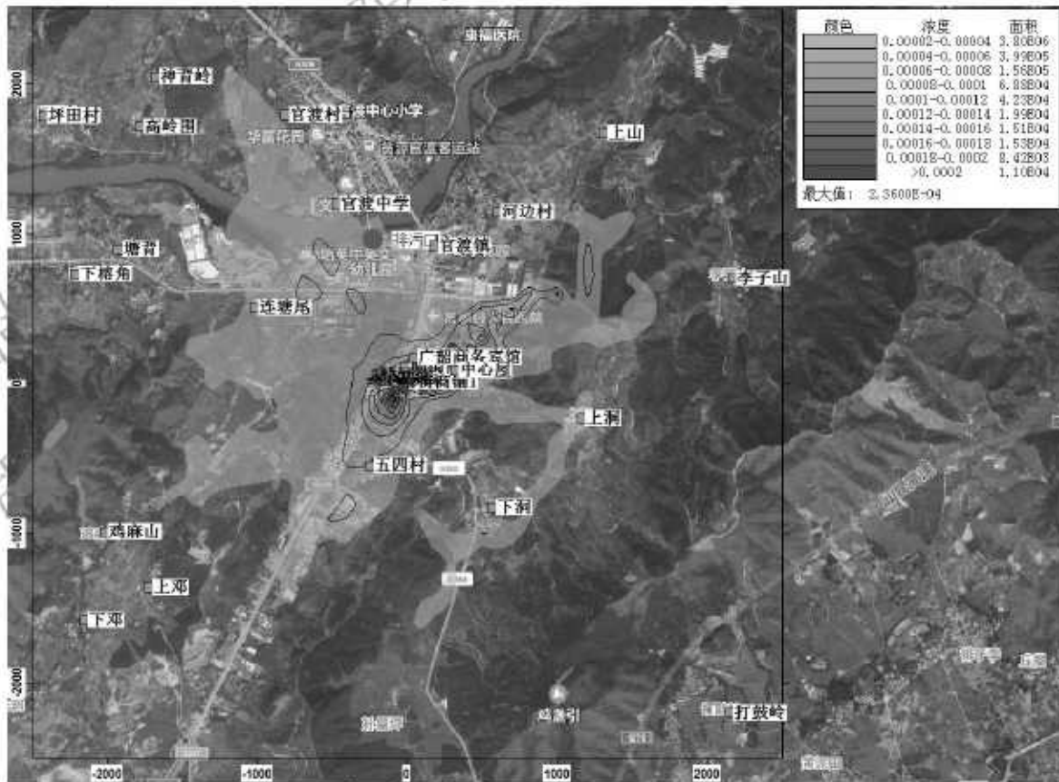
图 5-10 正常排放情况下 PM 2.5 日平均浓度最大值分布图
