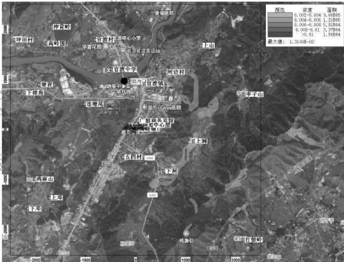
图 5-2 正常排放情况下 SO 2 小时平均浓度最大值分布图
