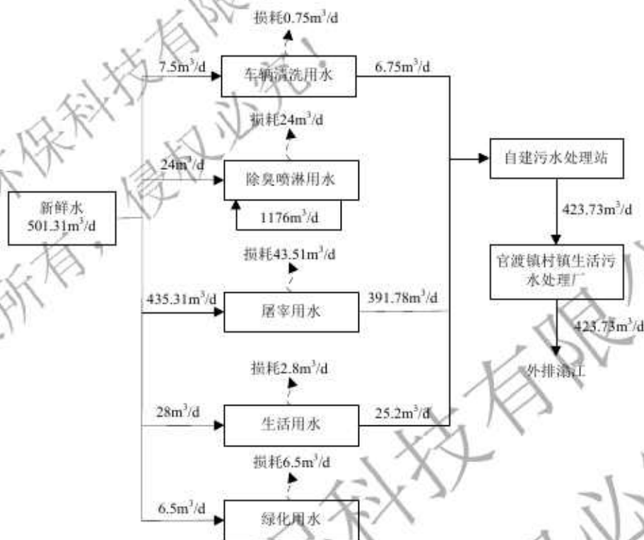
图 3-12 项目水平衡图
