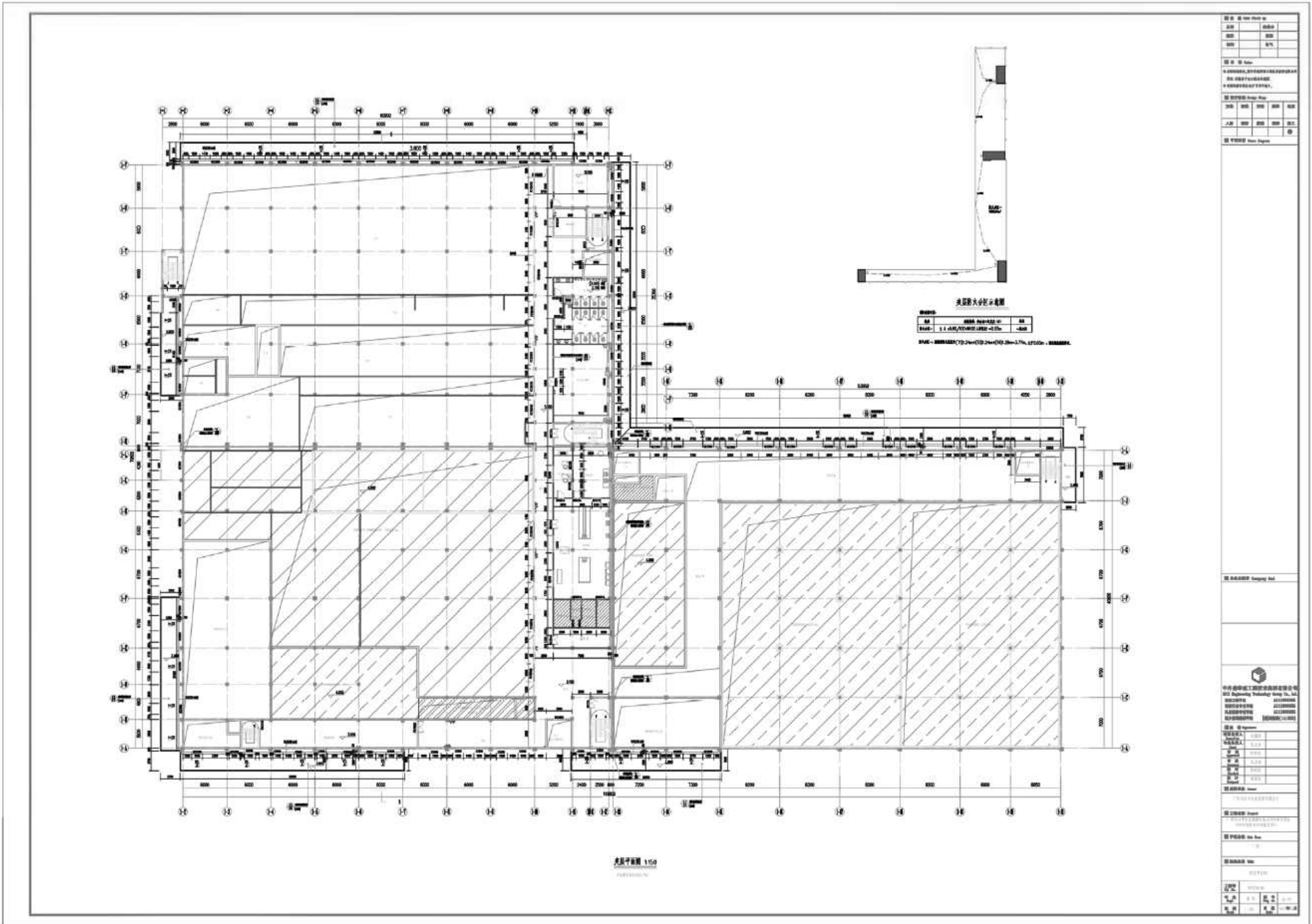
图 3-6 加工车间夹层平面布置图
