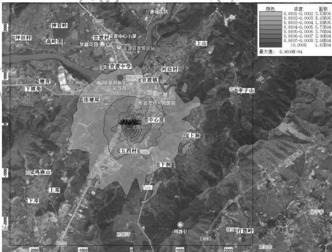
图 5-13 正常排放情况下 H 2 S 小时平均浓度最大值分布图
