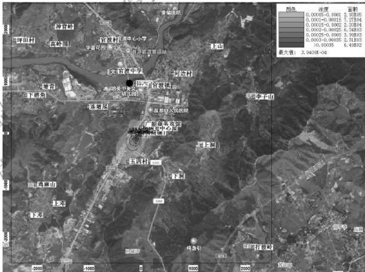
图 5-4 正常排放情况下 SO 2 年平均浓度最大值分布图
