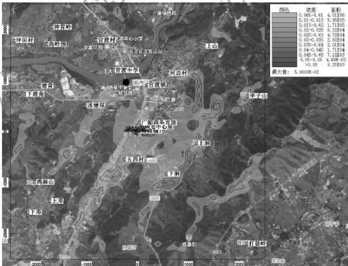
图 5-5 正常排放情况下 NO 2 小时平均浓度最大值分布图
