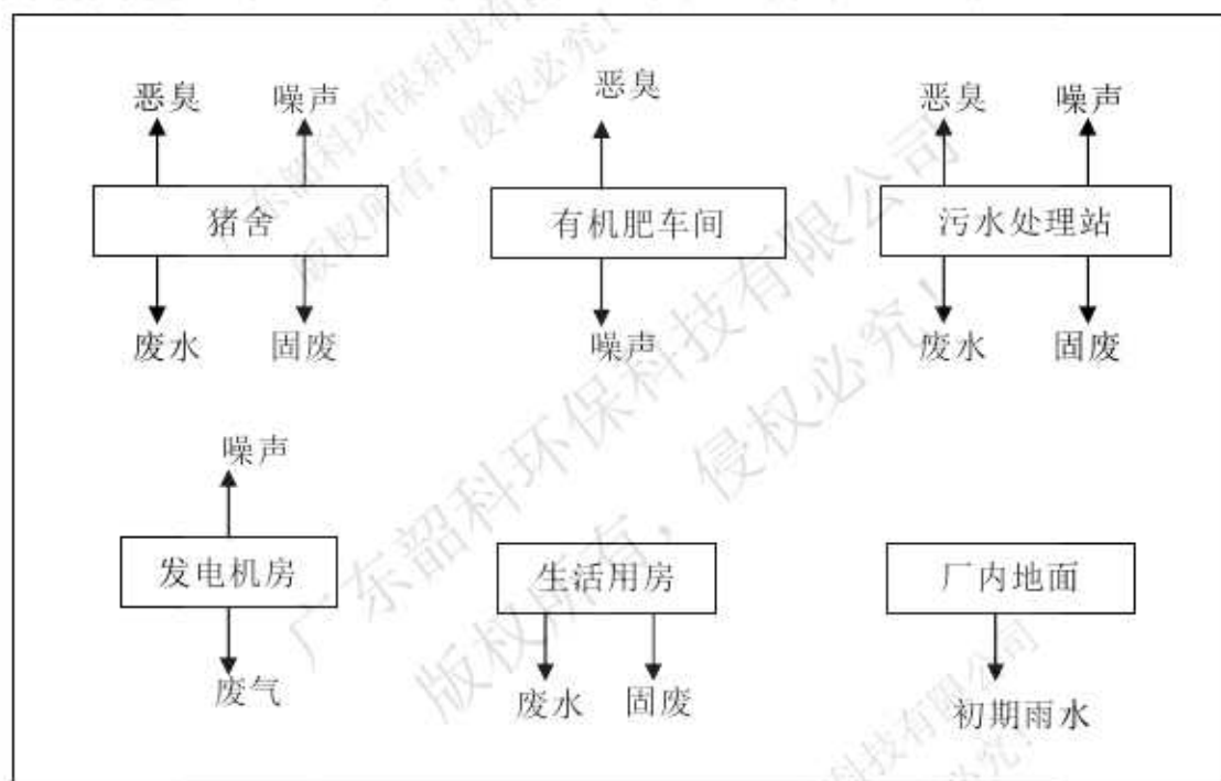
图 4-5 改扩建项目产污环节图
