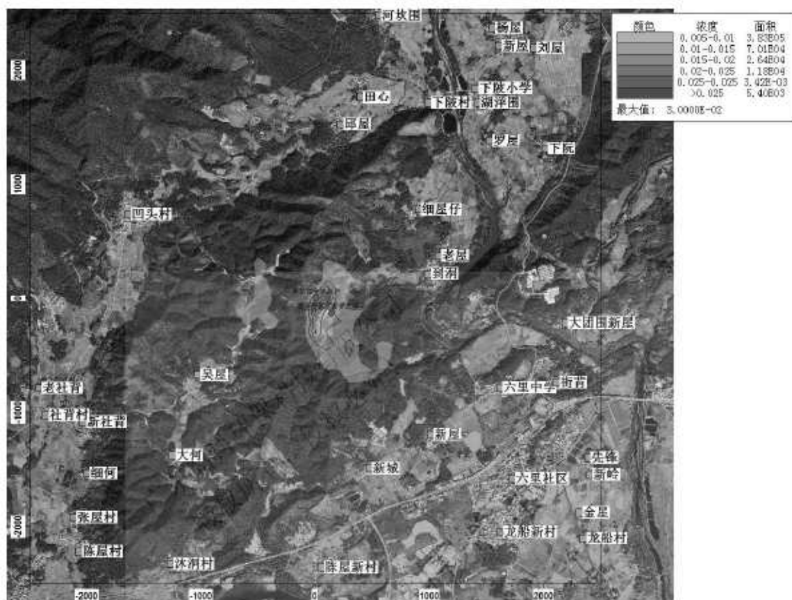
图 6-6 非正常排放情况下新增污染源 \text{NH}_3 小时平均浓度最大值分布图
