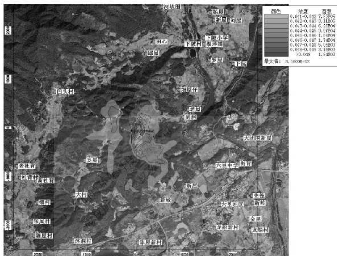
图 6-4 正常排放情况下叠加环境质量现状浓度后 \text{NH}_3 小时平均浓度最大值分布图
