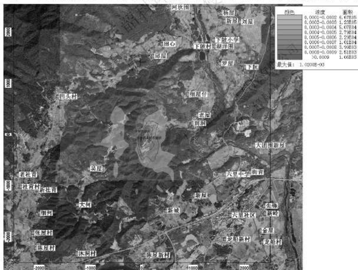
图 6-5 正常排放情况下叠加环境质量现状浓度后 \text{H}_2\text{S} 小时平均浓度最大值分布图
