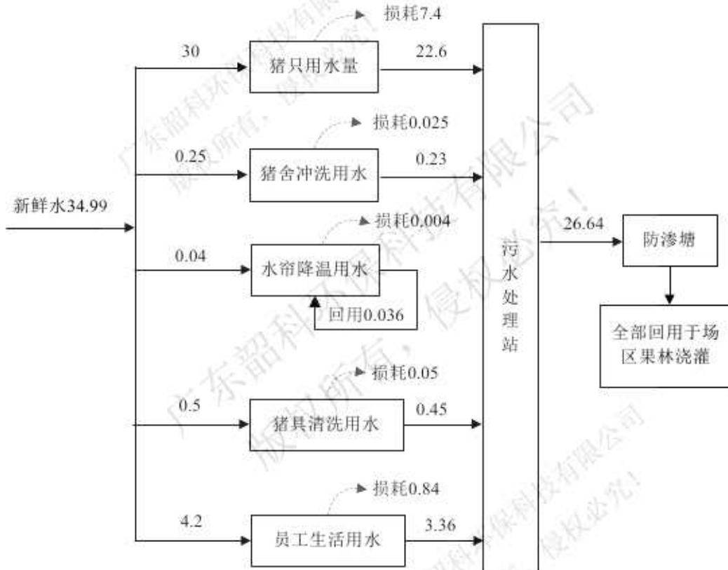
图 3-2 项目水平衡图（单位：m 3 /d）
