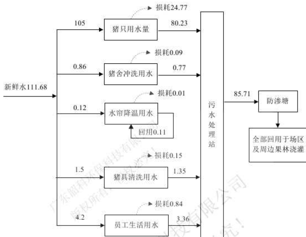
图 4-4 改扩建项目完成后水平衡图 (单位: m³/d)
