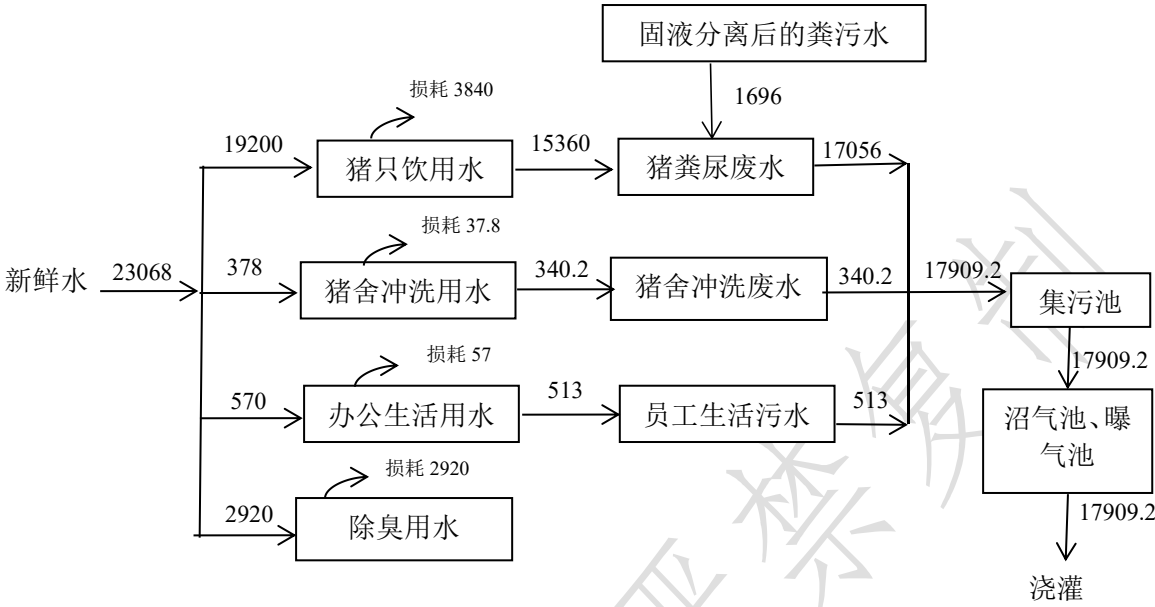
图 3-6 水平衡图（单位：m³/a）
