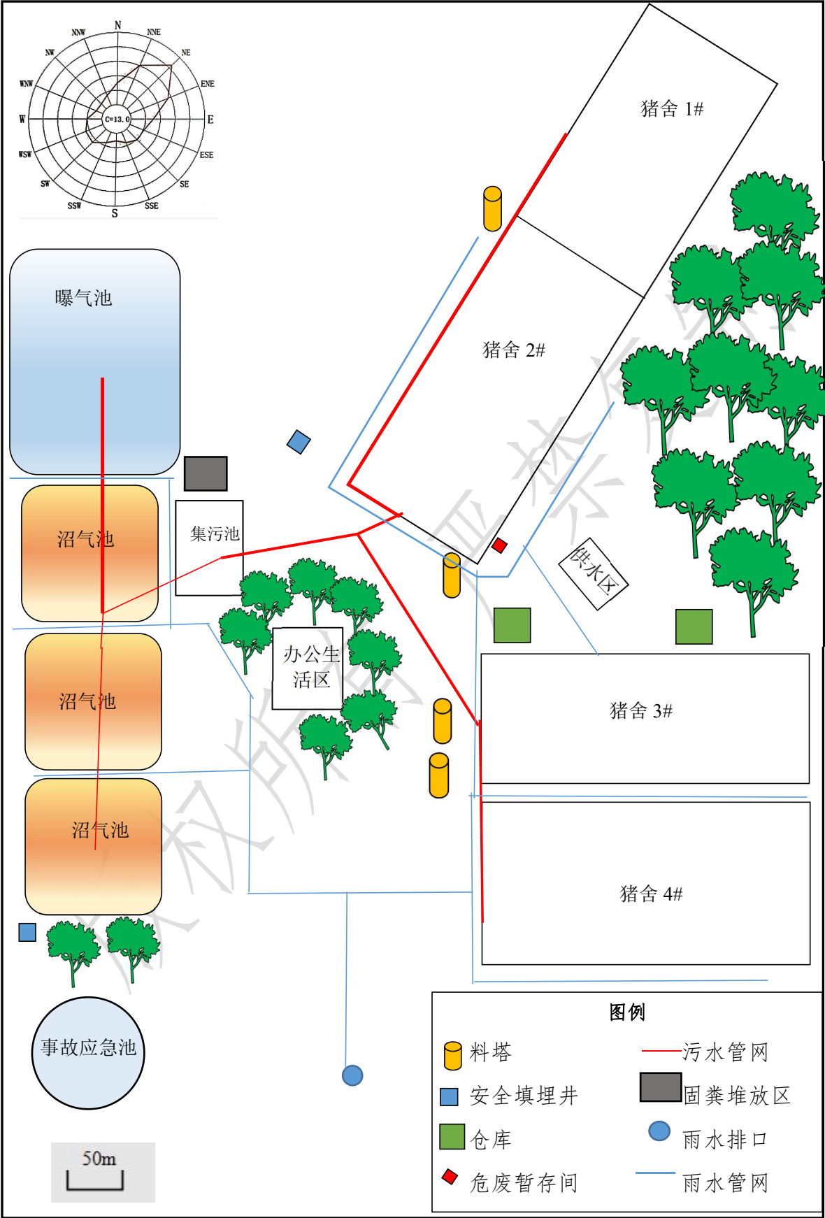
图 3-2 项目平面布置及雨污管网图
