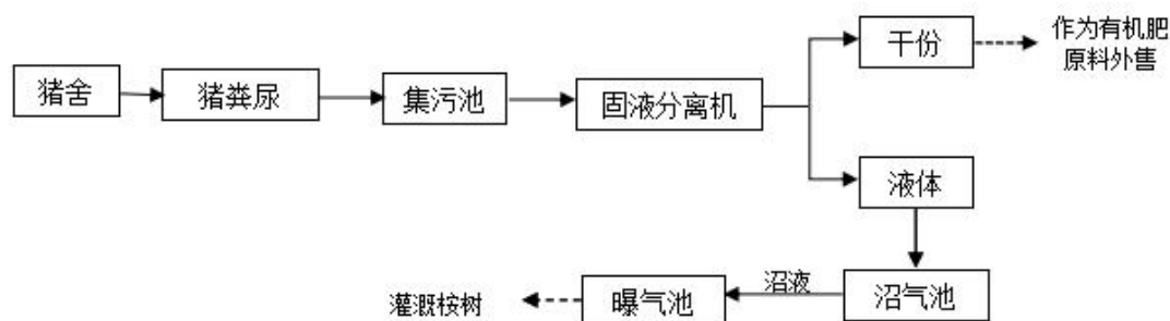
图 3-4 清粪及粪污处理工艺流程图
