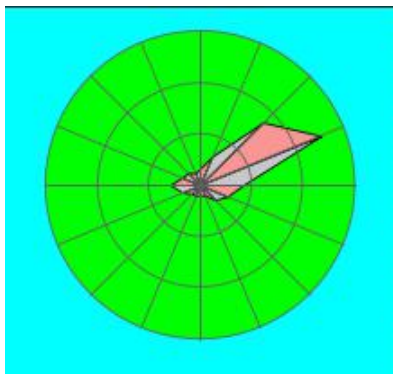
图 6-1 翁源县气象站风向玫瑰图 (统计年限: 2000-2020)
