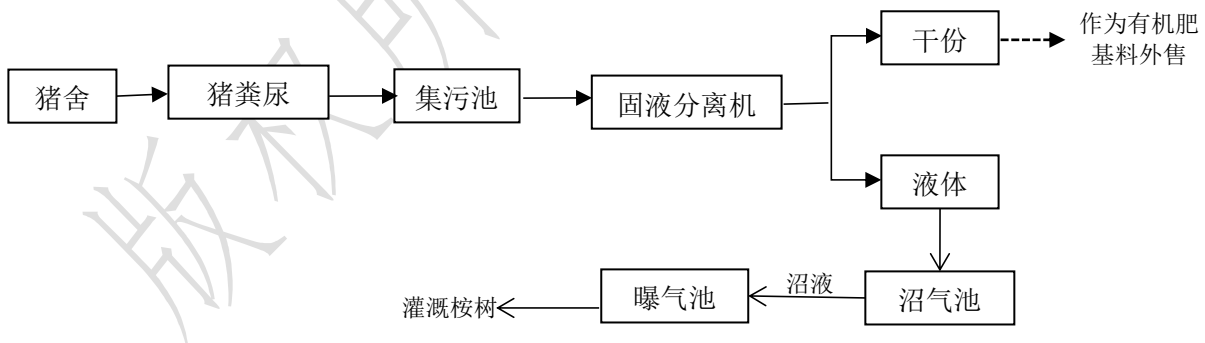
图 3-7 废水处理工艺流程图
