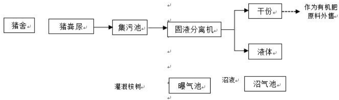
图 7-1 废水处理工艺流程图
