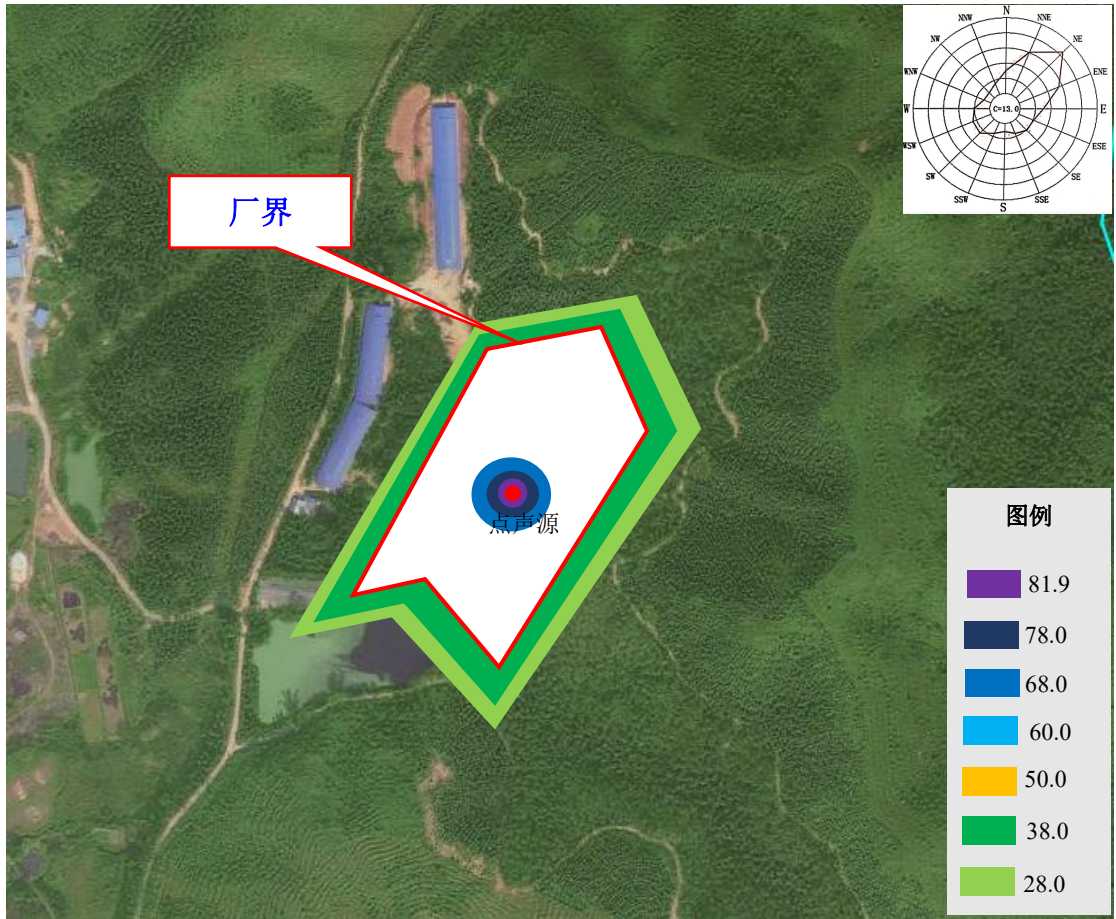
图 6-5 项目夜间噪声贡献值等值线图（单位：dB（A））
