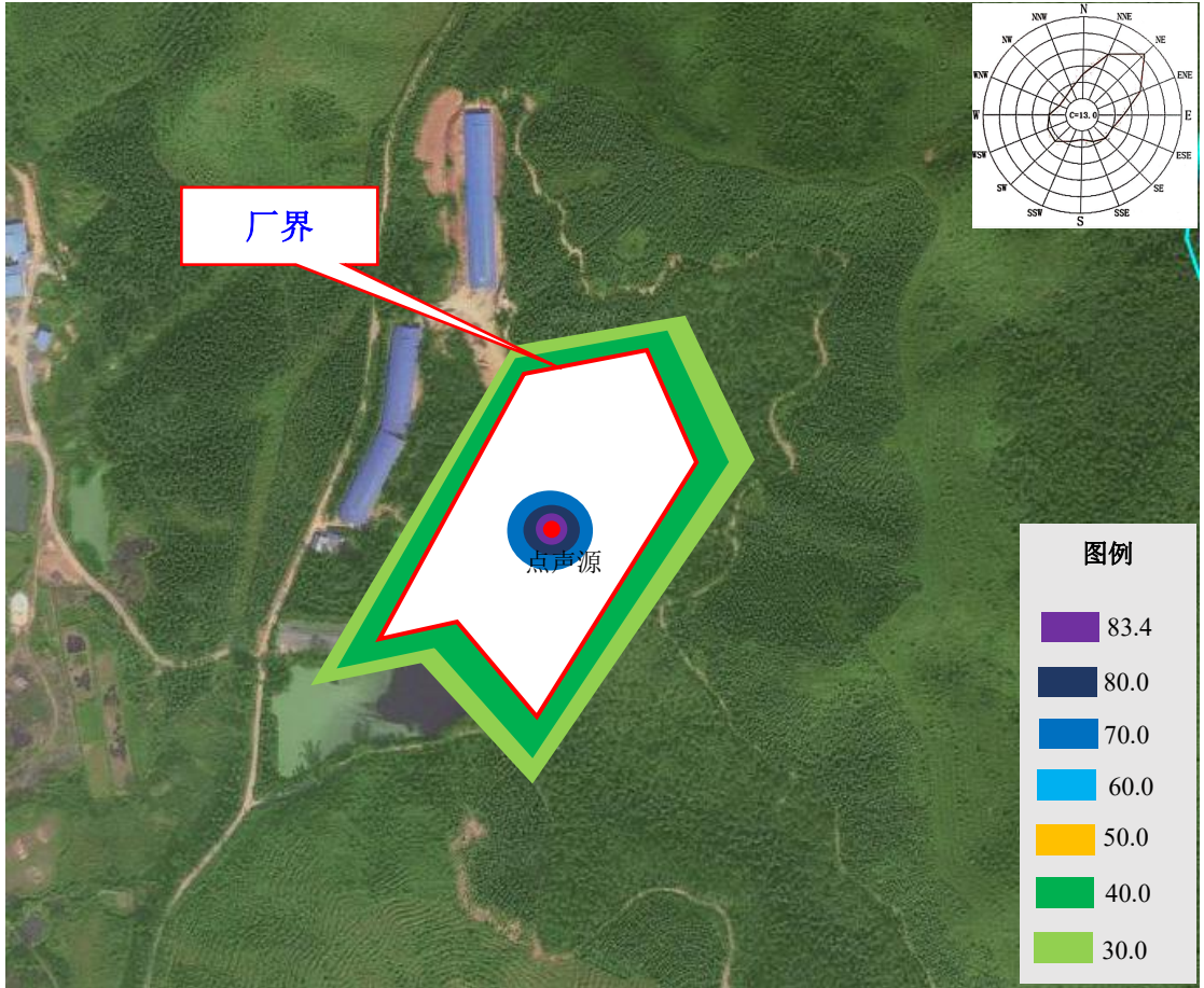
图 6-4 项目昼间噪声贡献值等值线图（单位：dB（A））
