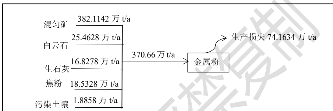
图 2-2 5号烧结机技改后物料平衡图
