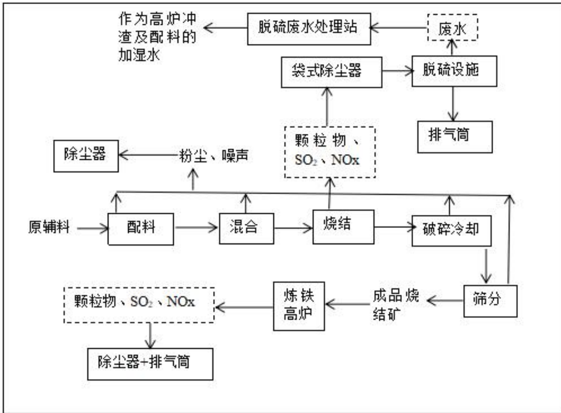
图 2-5 现有项目工艺流程图及产排污环节
