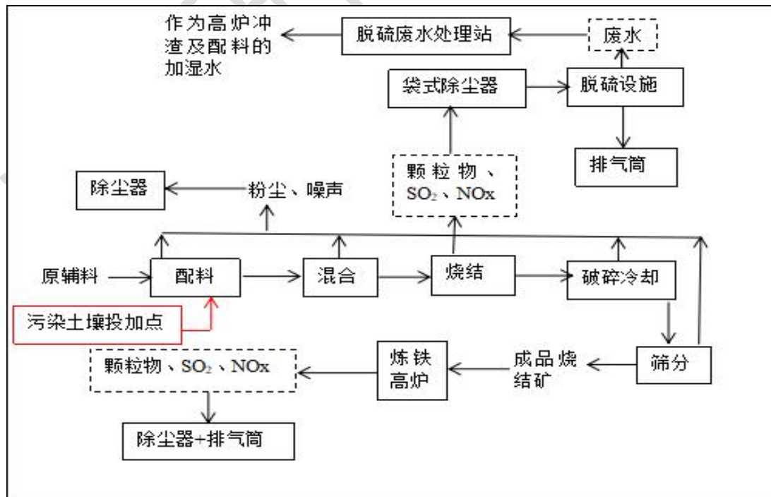
图 2-6 烧结+高炉协同处置污染土联合工艺流程图
