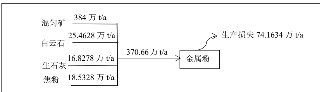
图 2-1 5号烧结机技改前物料平衡图
