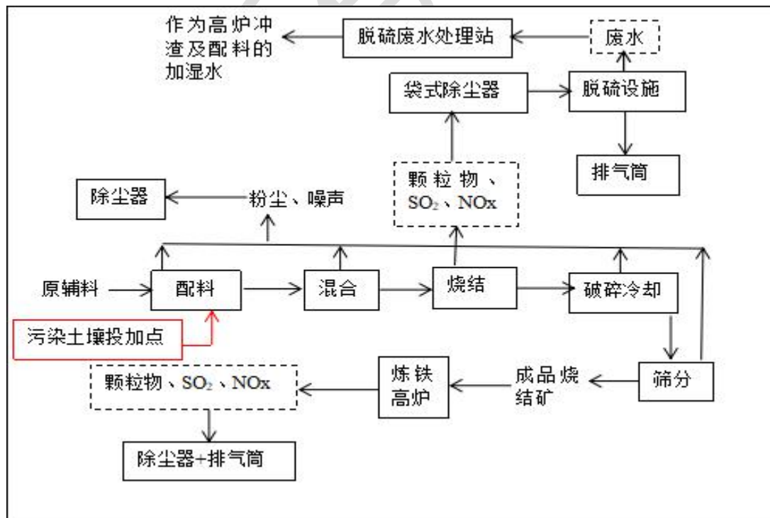
图 2.2-1 技改项目生产工艺及产污节点图
