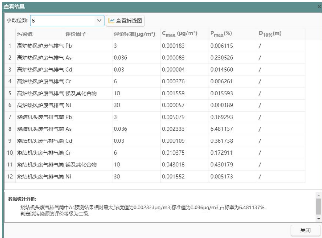
图 4.3-1 项目新增废气排放预测结果
