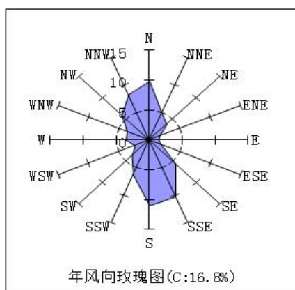
图 4.1-1 曲江气象站风玫瑰图（1999~2019 年）
