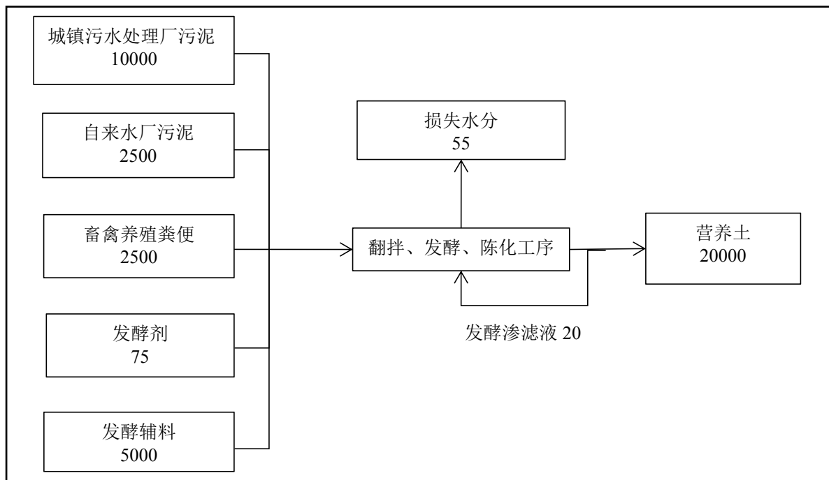
图 2-2 建设项目物料平衡图 （单位 t/a）
