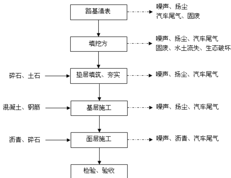
图 5-1 道路、停车场施工产污环节图
