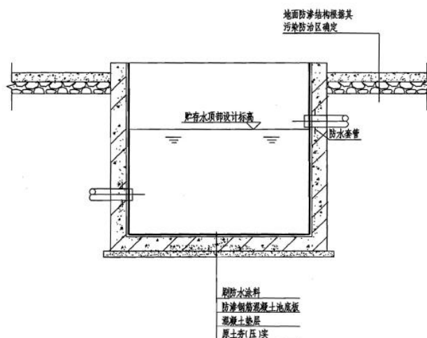
图 7-2 污水池防渗结构图
