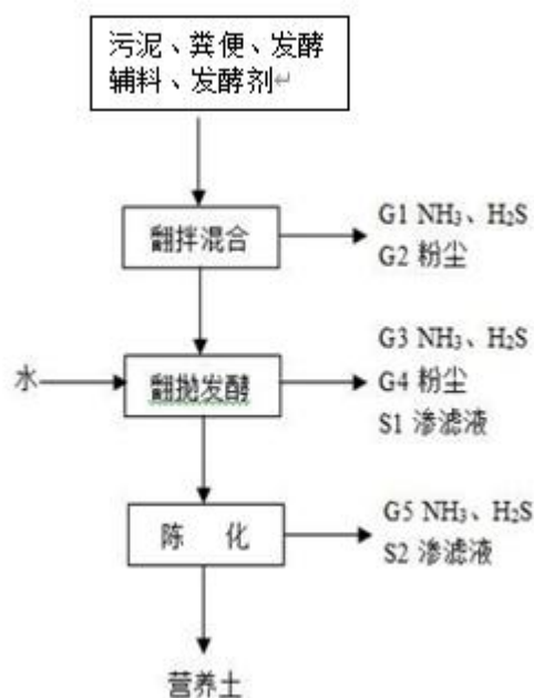
图 5-3 固废资源化处置工程主要生产工艺流程及产污环节图
