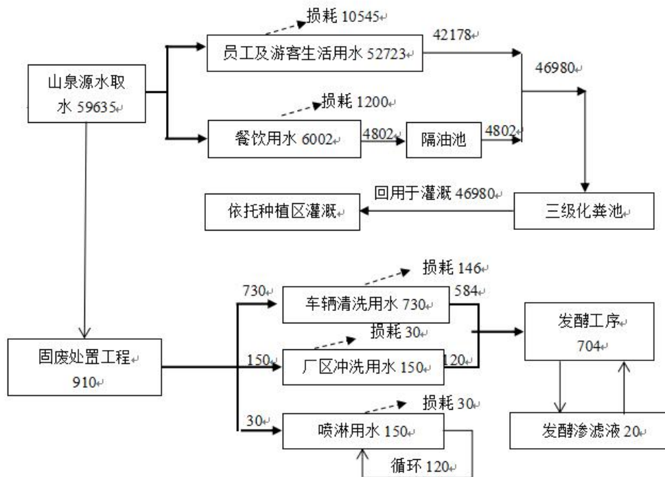
图 1-1 建设项目水量平衡图（单位 m³/a）
