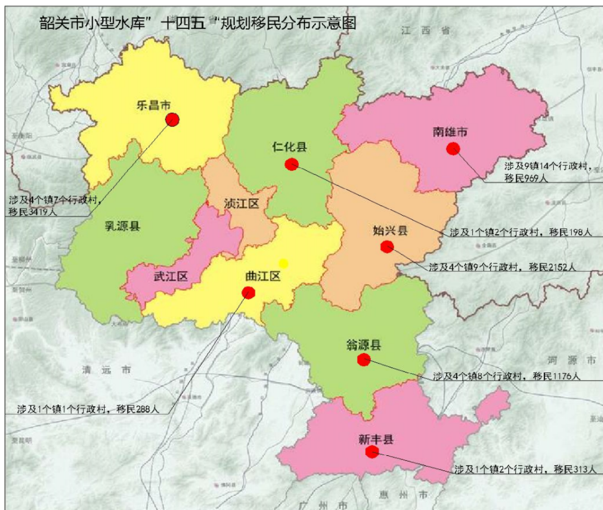
图 1.2-1 韶关市 2020 年小型水库移民人口分布示意图
