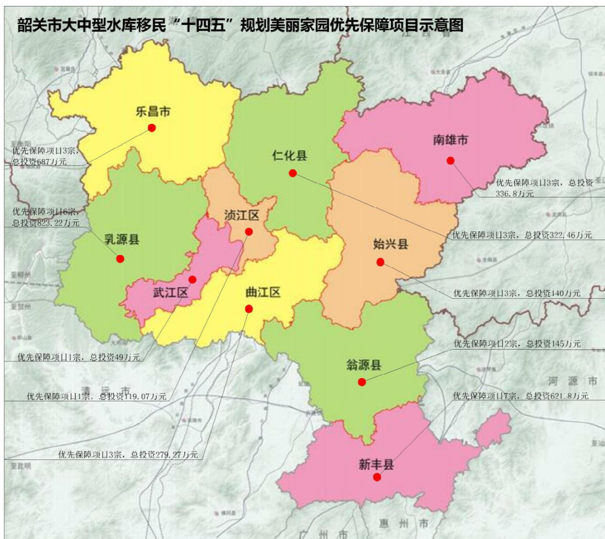
图 5.6-1 韶关市大中型水库移民后期扶持“十四五”规划美丽家园优先保障项目示意图
