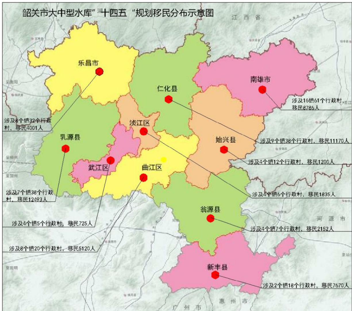
图 1.2-1 韶关市 2020 年大中型水库移民人口分布示意图
