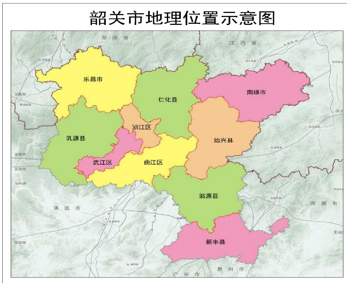
图 1.1-1 韶关市地理位置示意图
