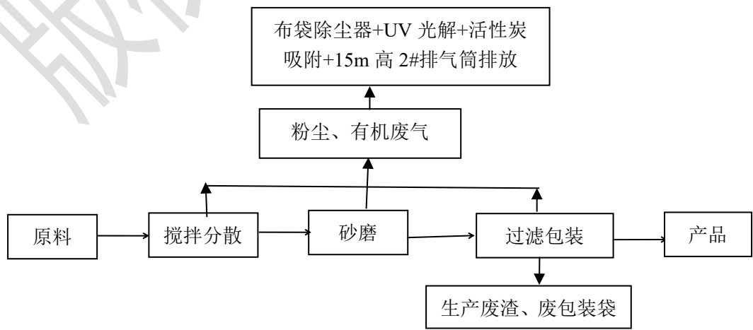
图 5-3 乳胶漆工艺流程及产污节点图
