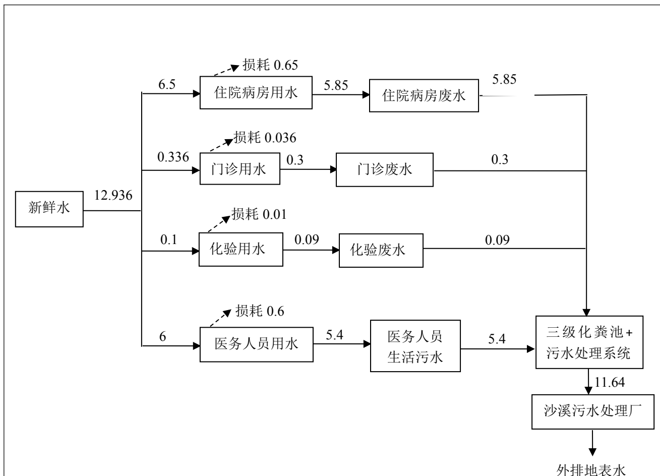
图 5-1 项目水平衡图 单位：m 3 /d
