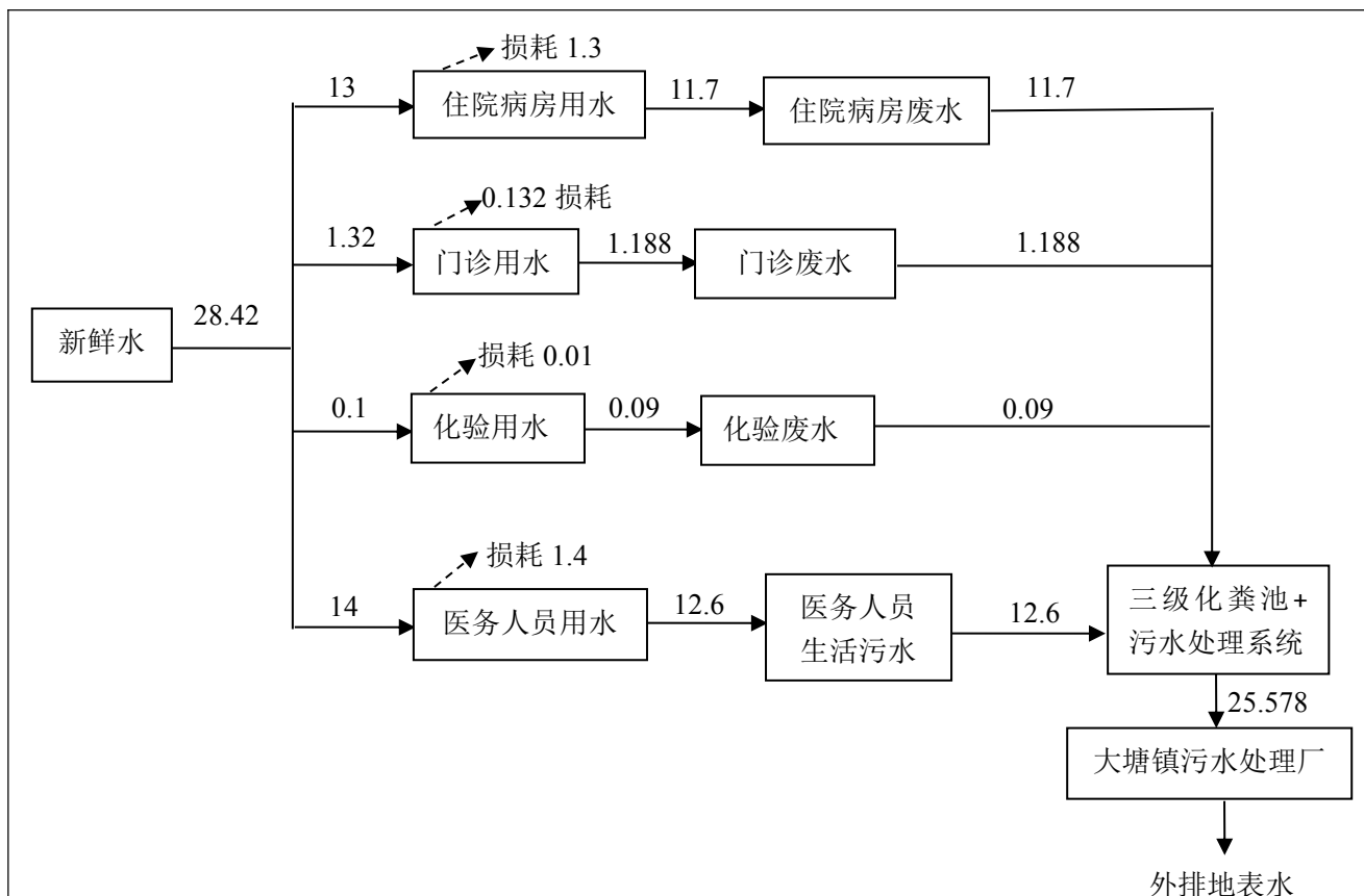
图 5-1 项目水平衡图 单位: m 3 /d
