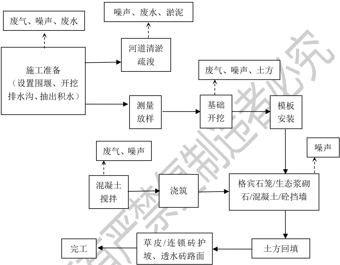
图5-1 施工工艺流程及产污节点图
